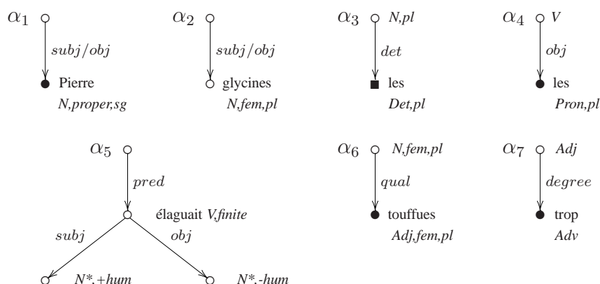
FIG. 4 – Arbres élémentaires. La flèche indique une relation de dépendance entre deux éléments, représentés par des nœuds. Pour l'ancre lexicale le nœud est annoté par un élément lexical. Les italiques indiquent des valeurs de traits. Les nœuds noirs et blancs indiquent des éléments saturés et non saturés, respectivement. Le nœud carré indique un translatif.
