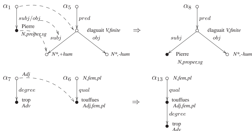
FIG. 5 – Mécanisme d’adjonction pour un dépendant valenciel (en haut) et pour un dépendant non valenciel (en bas).
