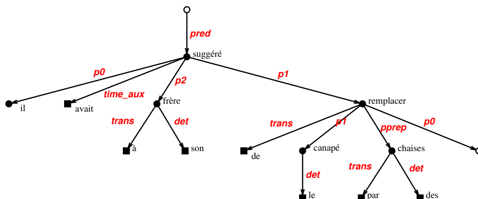
FIG. 1 – Analyse pour l'énoncé Il avait suggéré à son frère de remplacer le canapé par des chaises illustrant l'arbre de dépendance, les fonctions syntaxiques associées aux relations, les translatifs pour l'auxiliaire de temps, pour les déterminants, pour les prépositions et la proposition infinitive. p0 , p1 , p2 et pprep indiquent respectivement le sujet, l'objet, l'objet indirect et un complément prépositionnel.
