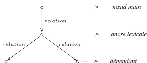
FIG. 3 – Parties constitutives de l'arbre élémentaire. Les nœuds et relations au-dessous de l'ancre lexicale ne sont présents que si l'ancre présente des dépendants valenciel.
