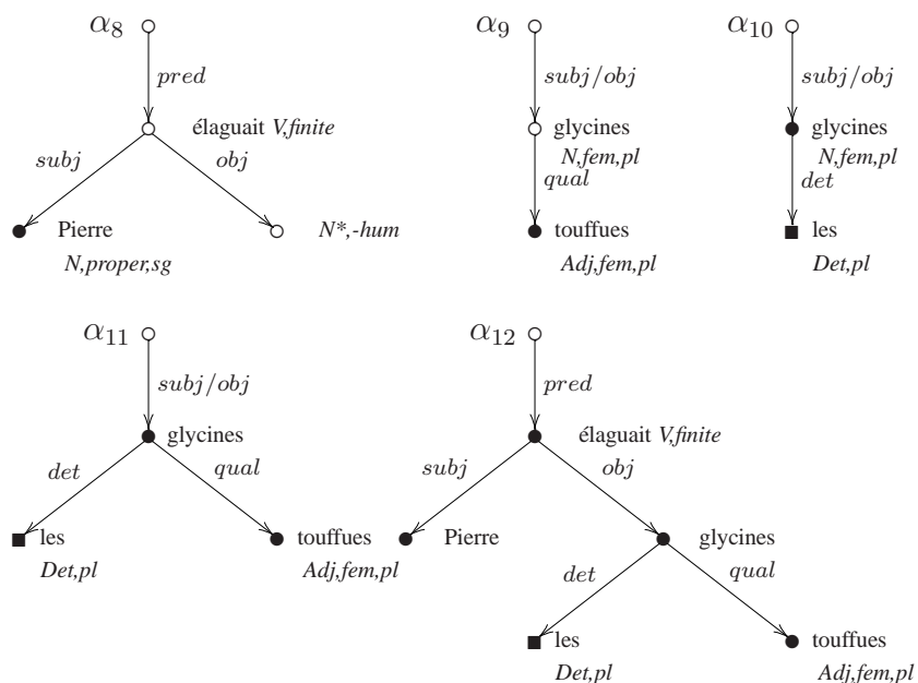
FIG. 6 – Arbres dérivés
