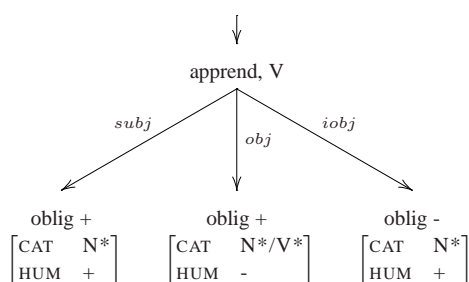
FIG. 2 – Cadre de valence représenté comme une arbre de dépendance. Le trait oblig indique la nature obligatoire ou facultatif du terme. N* et V* indiquent un nœud structural à tête nominale (nom commun, nom propre, pronom), ou verbale (complétive, proposition infinitive), respectivement.
