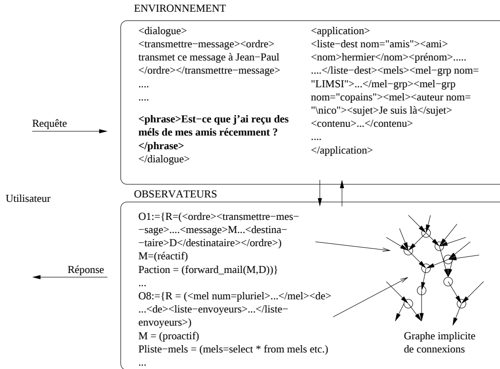
FIG. 1 – Fonctionnement général du système d'analyse d'InterViews. Exemple de traitement sur des objets de haut niveau, ici des listes de mels.
