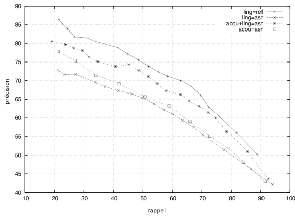
Fig. 1: Performance de la détection de segments spontanés (degré de 4 à 10) en fonction d'un seuil sur le score de classification
