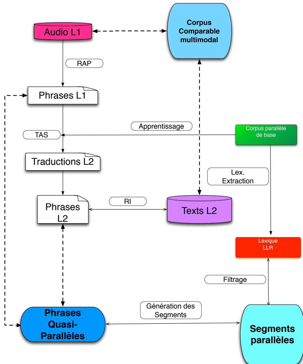
FIGURE 5.10 – Principe du système d'extraction des segments parallèles avec la méthode SentExtract + LLR_lex .
