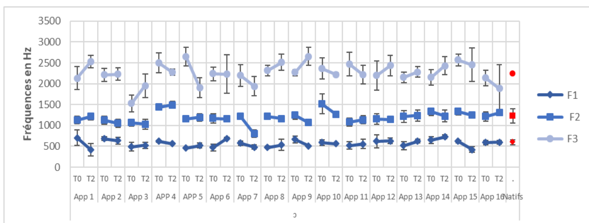
Figure 72 : Valeurs formantiques moyennes en Hz et écarts types des /ɔ/ produits par les apprenants à T0 et T2 (en bleu) et des /ɔ/ par les natifs (en rouge).
