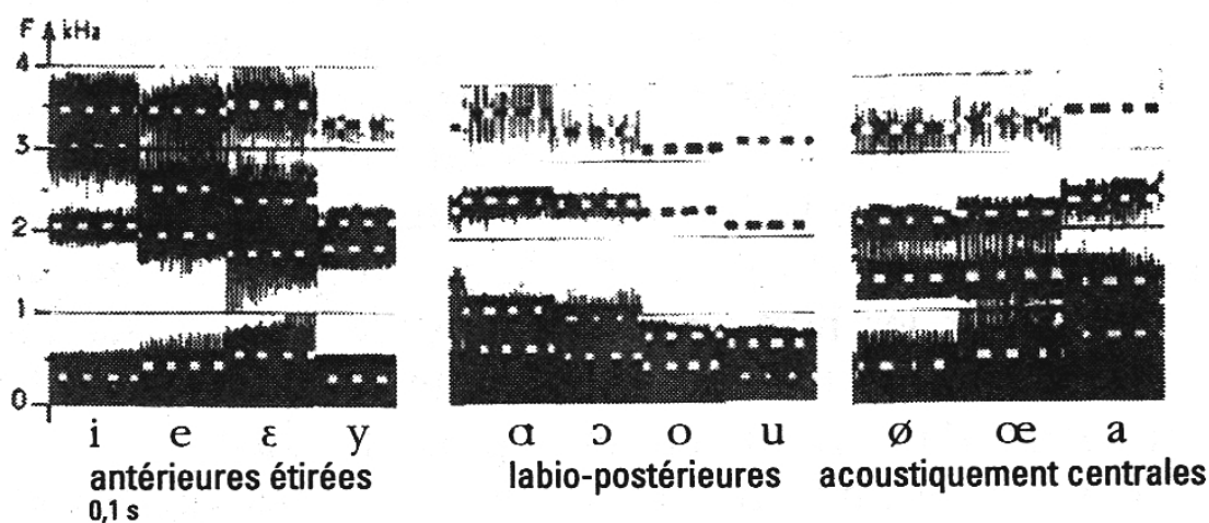
Figure 16 : Spectrogramme des voyelles orales du français. D'après Liénard (1977) extraite de Vaissière (2006 : 72).
