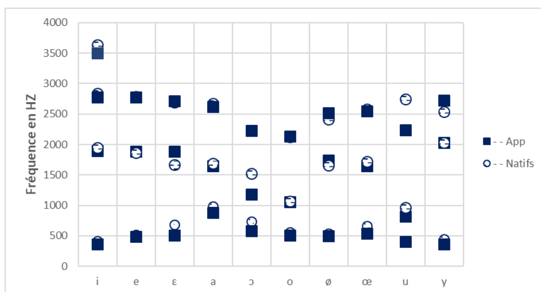
Figure 39 : Valeurs formantiques moyennes (F1, F2, F3) et F4 pour /i/ en Hz des voyelles cibles produites par nos 16 apprenants (carré plein) et par les natifs (rond discontinu).
