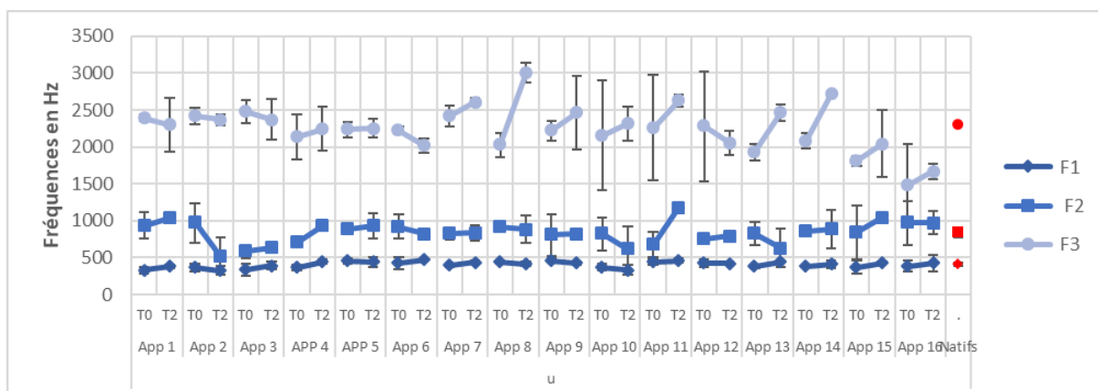
Figure 70 : Valeurs formantiques moyennes en Hz des /u/ réalisés par chaque apprenant à T0 vs. T2, en bleu (moy de 4 réalisations par apprenant) et par les natifs, en rouge (tous confondus).
