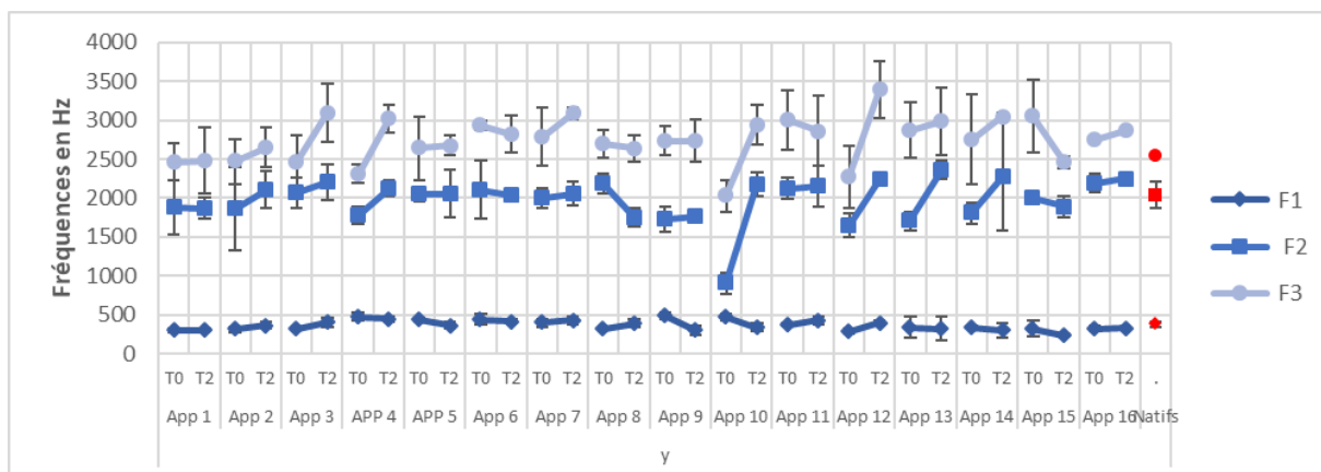
Figure 67 : Valeurs formantiques moyennes en Hz des /y/ réalisés par chaque apprenant à T0 vs. T2, en bleu (moy de 4 réalisations par apprenant) et par les natifs, en rouge (tous confondus).
