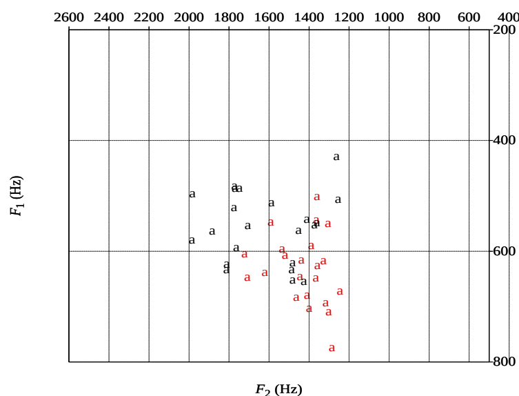
Figure 19 : distribution sur les axes F1/F2 de la voyelle /a/ du dialecte tunisien, parler de Sousse produite par 10 locutrices natives en contexte [-post] en noir et en contexte [+post] en rouge.
