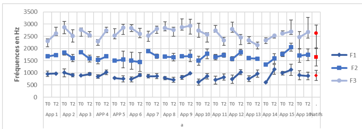
Figure 66 : Valeurs formantiques moyennes en Hz des /a/ réalisés par chaque apprenant à T0 vs. T2, en bleu (moy de 4 réalisations par apprenant) et par les natifs, en rouge (tous confondus).
