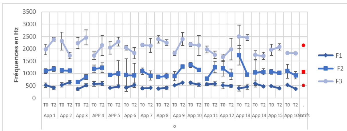
Figure 71 : Valeurs formantiques moyennes en Hz et écarts types des /o/ produits par les apprenants à T0 et T2 (en bleu) et par les natifs (en rouge).
