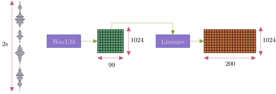
FIGURE 4.2 – Extraction de caractéristiques basée sur un modèle WavLM
