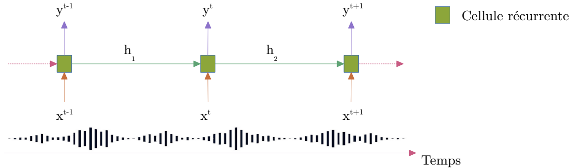
FIGURE 2.3 – Fonctionnement d’un réseau récurrent générique avec des entrées x , des sortie y et un historique h
