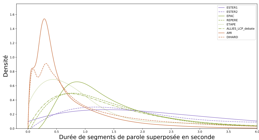
FIGURE 3.2 – Distribution des durées des segments de parole superposée par corpus
