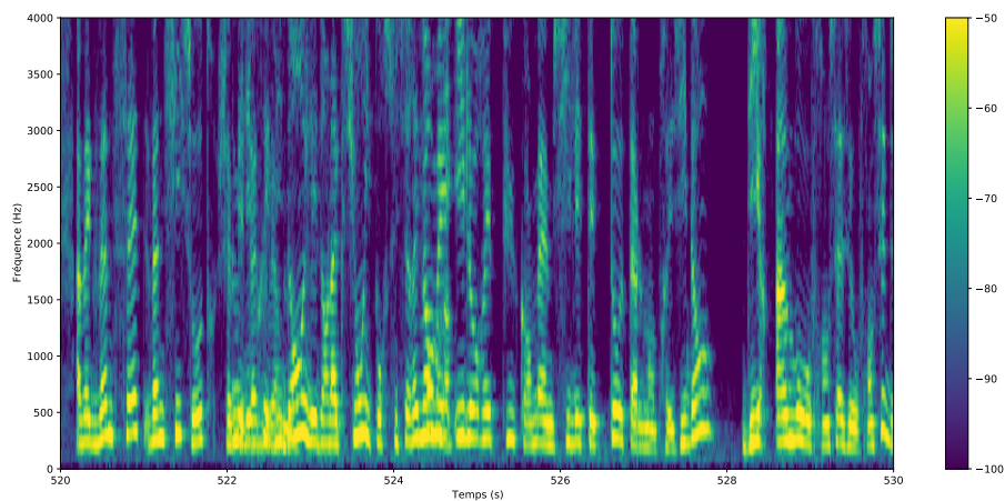
FIGURE 2.6 – Exemple d'un spectrogramme de parole
